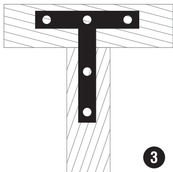
3 Placa de unión T
