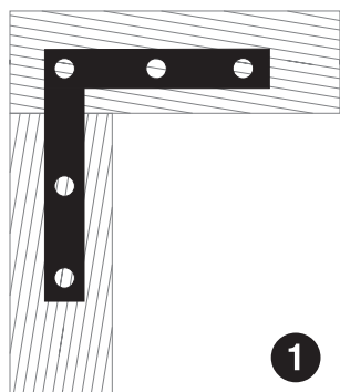
1 Refuerzo de unión L
